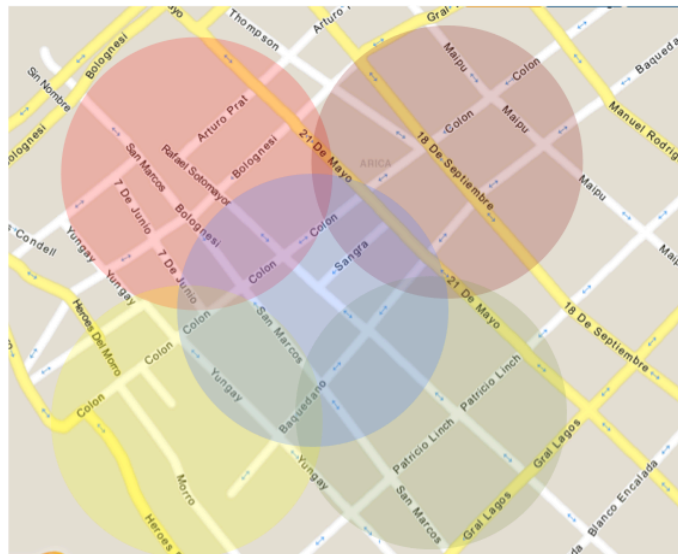
Ampliación de la capacidad de tráfico mediante nuevas estaciones base Figura A1.9
