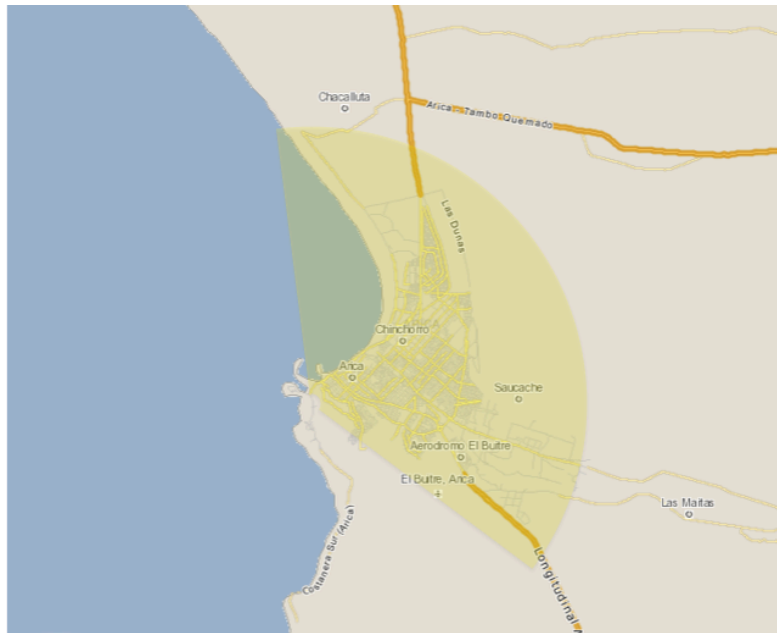
Cobertura teórica en Arica con una sola estación base sobre el Morro
